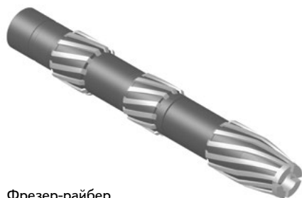
Фрезер-райбер типа ФРЛ
